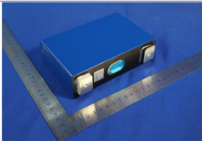
图 3 电芯侧面 Picture 3 Side view of cell
